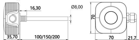
Размеры датчика, мм
