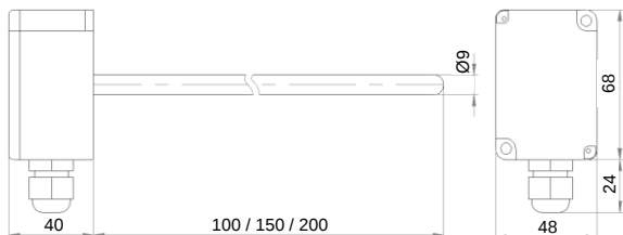
Размеры датчика, мм
